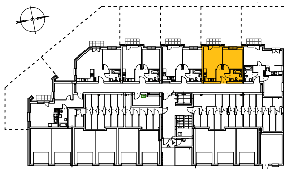
RZUT PARTERU
